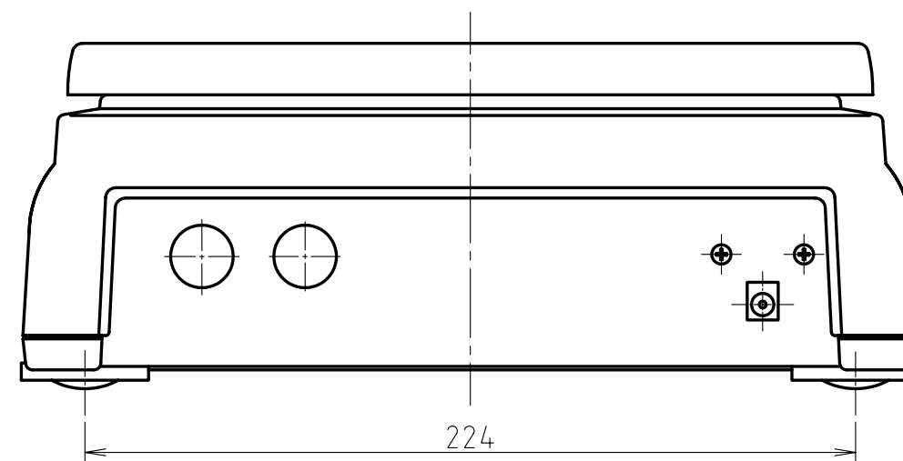
背面図
