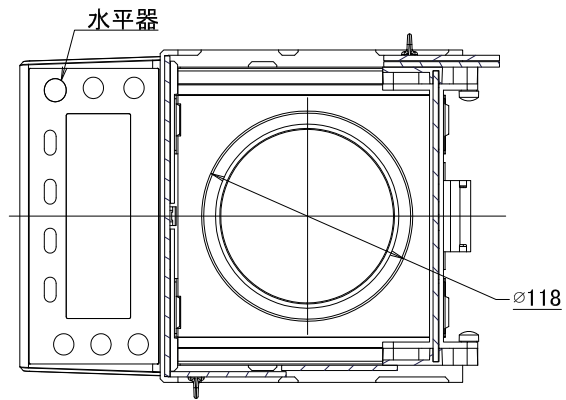
A-A (1 : 3)
